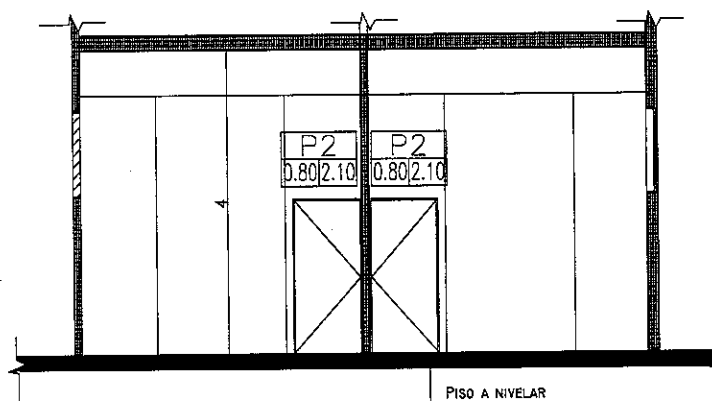
CORTE B-B READECUACION DE ESPACIO PARA CUATRO DEPOSITOS ESC. 1:100
