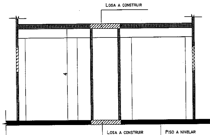
CORTE A-A READECUACION DE ESPACIO PARA CUATRO DEPOSITOS ESC. 1:100
