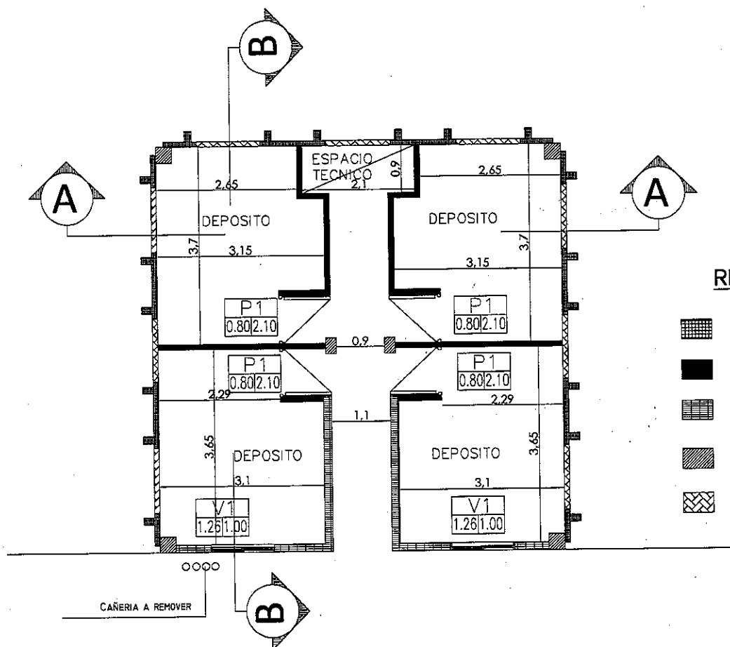
PLANTA DE ARQUITECTURA READECUACION DE ESPACIO PARA CUATRO DEPOSITOS ESC. 1:100
